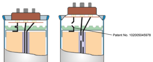
Prinzip der Überdruck-Abreißsicherung
