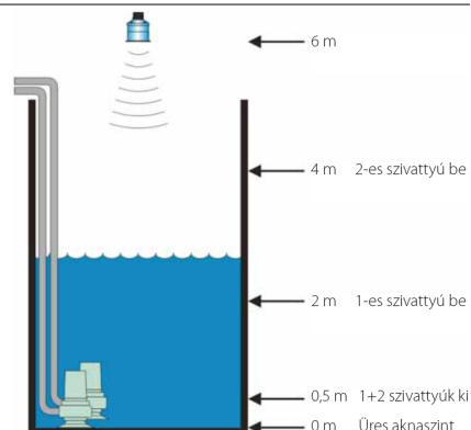
Váltott rásegítő üzemmódban működő szivattyúk elvi ábrája
