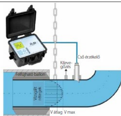
A mérőrendszer elvi beépítési ábrája
