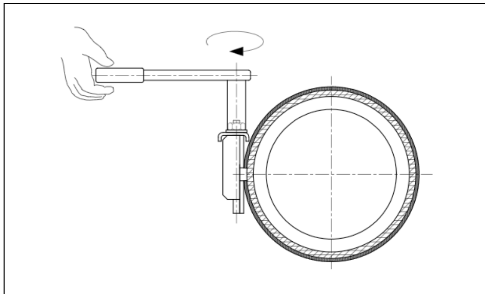
6-41 ábra Az anyák meghúzása
