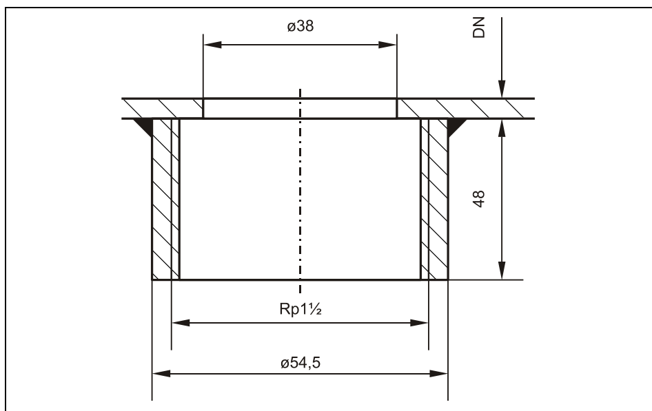
6-31 ábra Méretek hegeszthető csonk szerelése esetén
