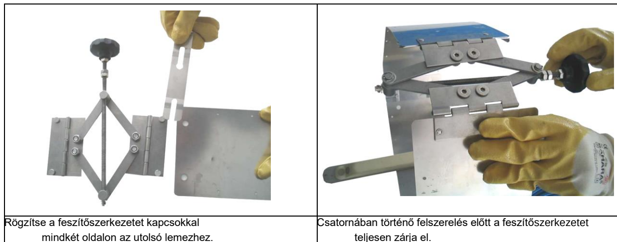
6-5 ábra RMS2 rögzítőrendszer összeszerelése
