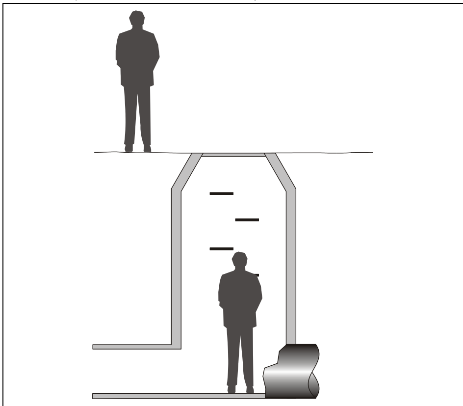
6-24 ábra Beépítés 1. lépés: két személy a szereléshez
