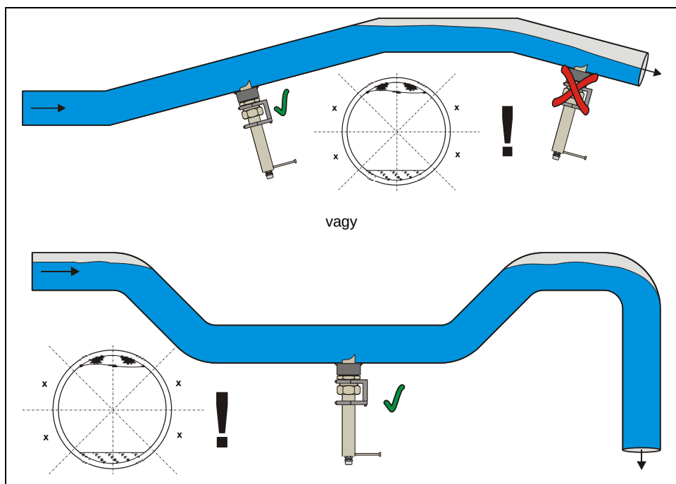
4-14 ábra Szifon jellegűen kialakított vízszintes csőszakasz
