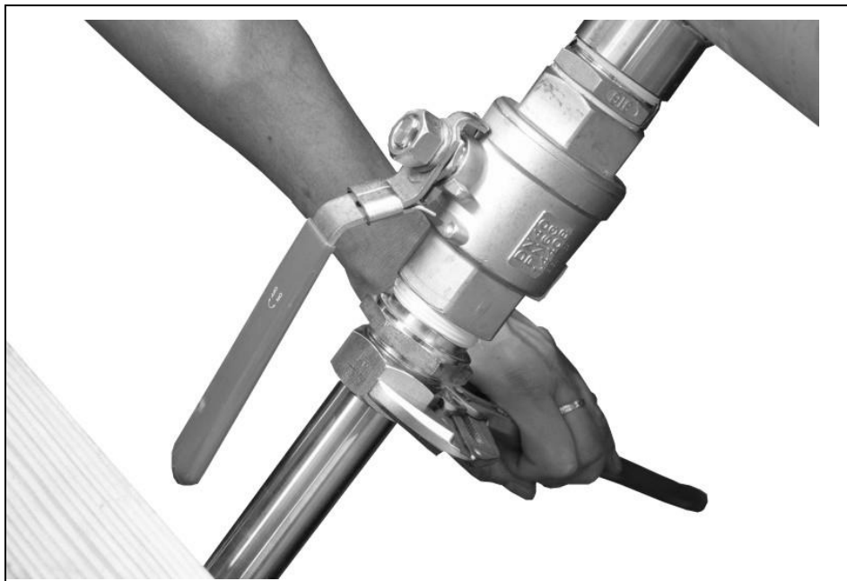
4-32 ábra Érzékelő rögzítése
