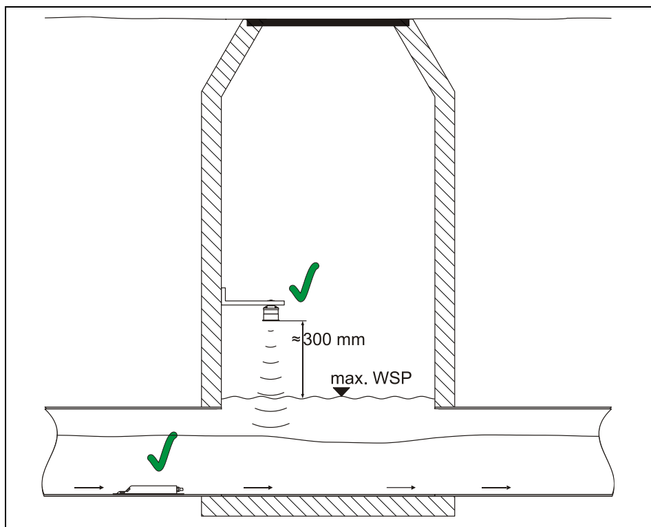
4-9 ábra Elhelyezés aknában legalább 150 mm telítettségi szint felett
