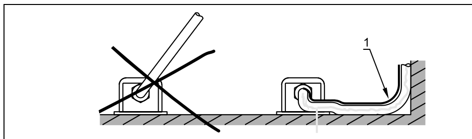
4-40 ábra Utasítások a kábelelvezetésre
