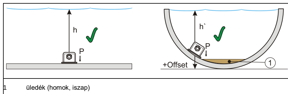
4-19 ábra Szerelés: Érzékelők integrált nyomásmérő cellával
