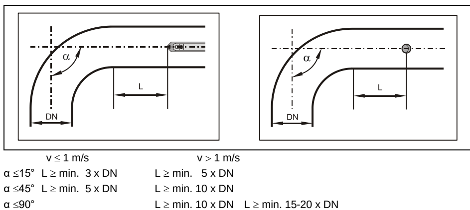
4-2 ábra Érzékelő elhelyezése kanyar vagy könyök után
