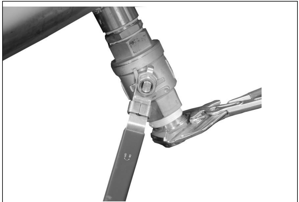
4-30 ábra Érzékelő tömítőidom felszerelése golyócsapra
