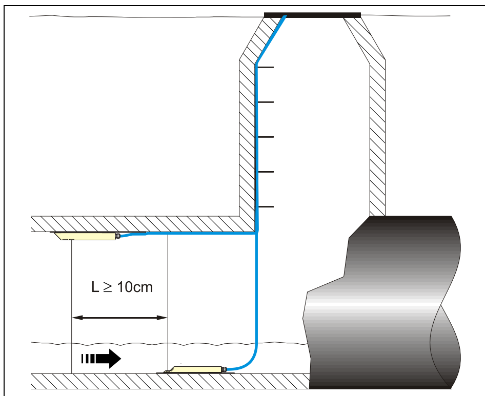
4-22 ábra Példa az érzékelők beépítésére
