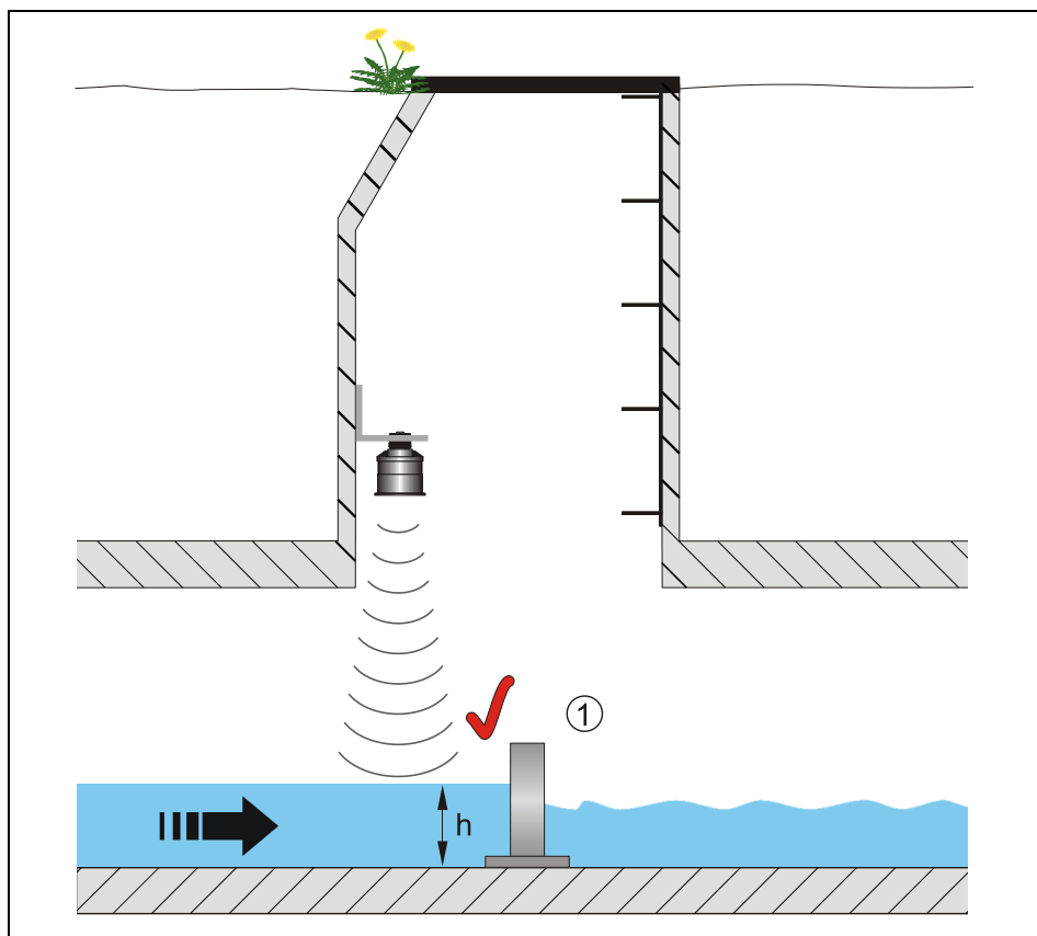
1 duzzasztó elem
