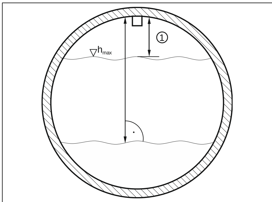
4-21 ábra Levegő ultrahangos szintérezékelő beépítése
