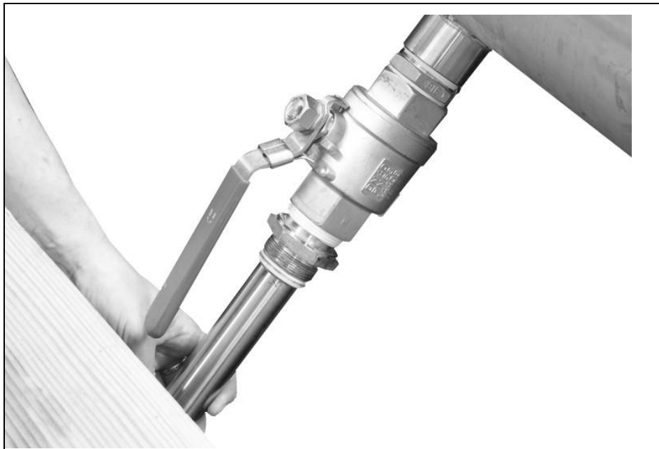
4-31 ábra Érzékelő pozicionálása
